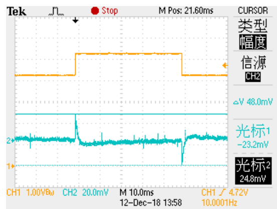
1 通道橙色线为输入, 2 通道蓝线为输出
