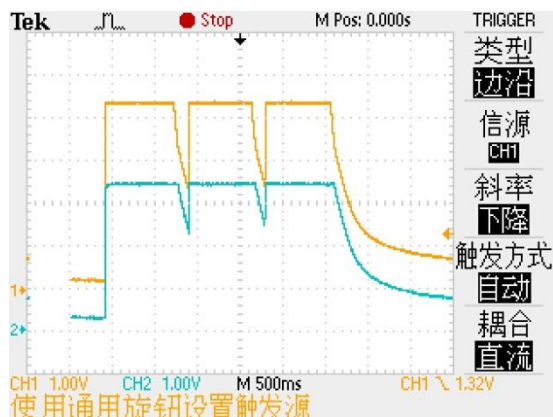
1 通道橙色线为输入, 2 通道绿线为输出
